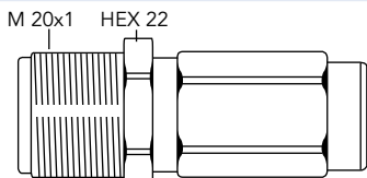
3,5/12f-XX
