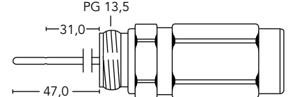
PG13,5m-XX
